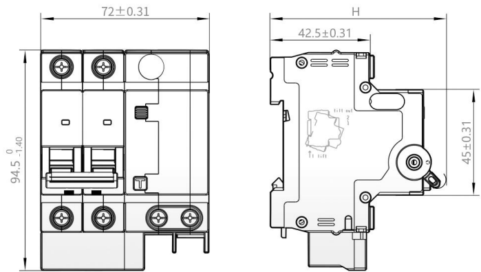
图 3 外形及安装尺寸
