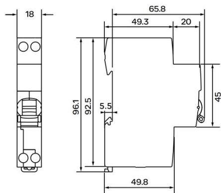
图 3 外形及安装尺寸
